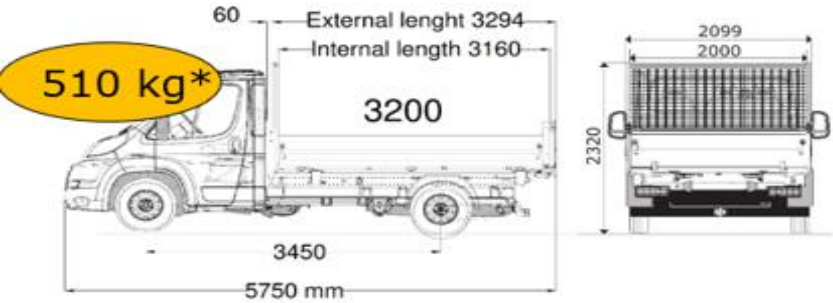
L2 Chassis Cab : 3200 tipper
